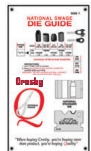
National Swage Die Guide
