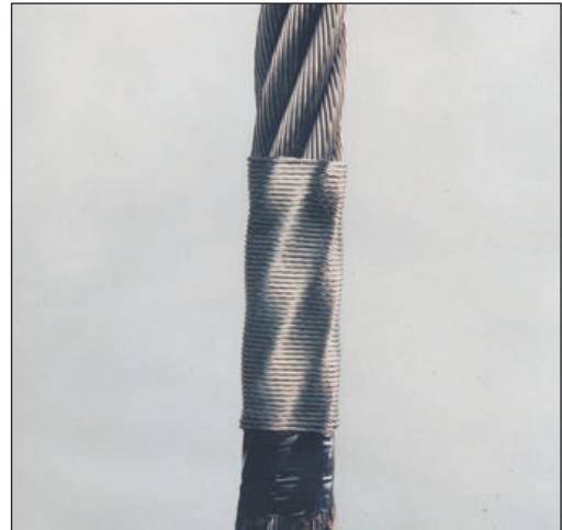
Seizing of Wire Rope
