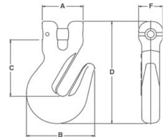
A-1358 Grab Hook
